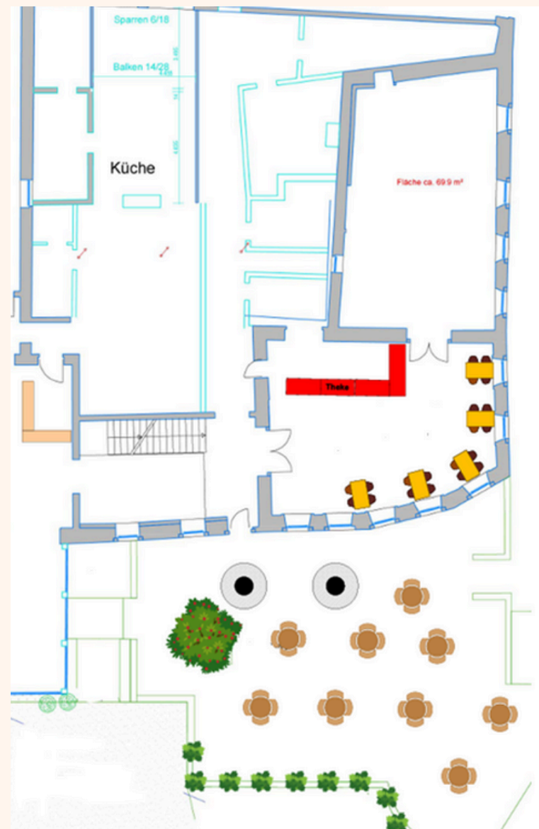
Erdgeschoss
